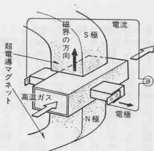
MHD発電の原理
